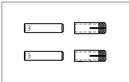
M8 Befestigungsset 266.050.005
